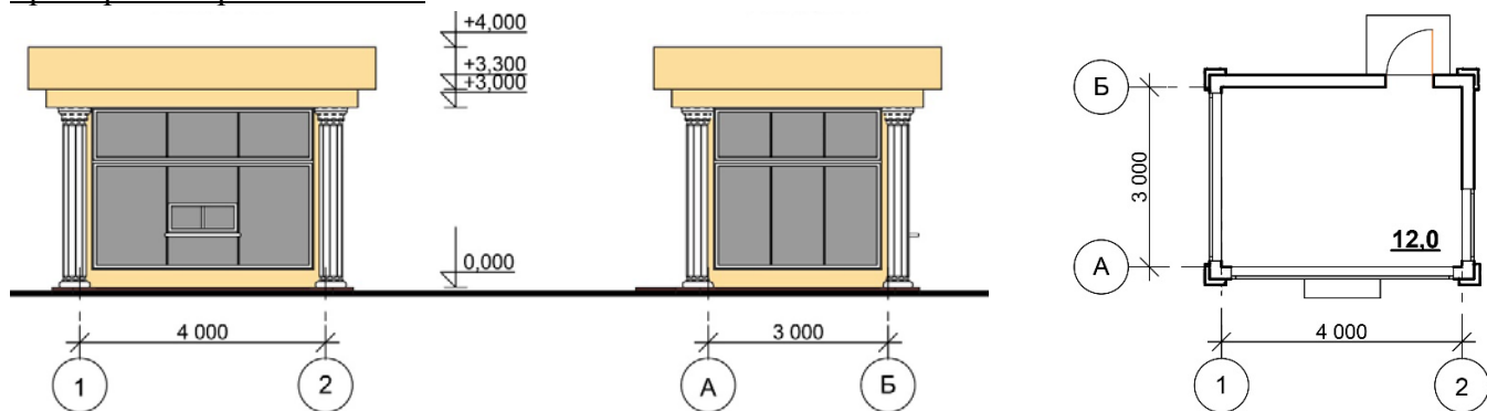
Рис. «Основные параметры места размещения нестационарного торгового объекта для киосков» схемы места размещения нестационарного торгового объекта при островном размещении киоска с тупиковым подходом:
