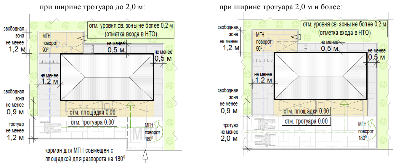
Рис. «Основные параметры места размещения нестационарного торгового объекта для киосков» схемы места размещения нестационарного торгового объекта при островном размещении киоска с тупиковым подходом:
