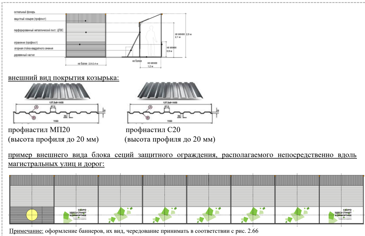
рис. 2.71 «внешний вид защитно-охранного (временного) ограждения ТИП 2»
