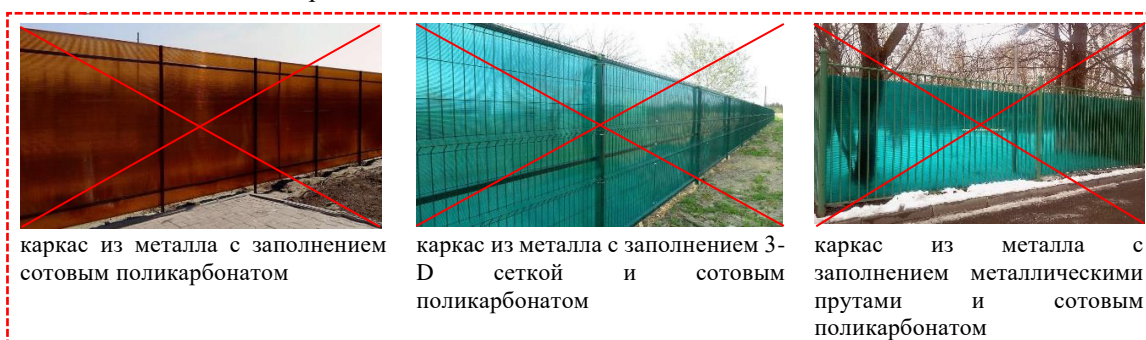
рис. 2.11 «пример внешнего вида заборов из поликарбоната, не допускаемых к размещению вдоль «вылетных» магистралей»
