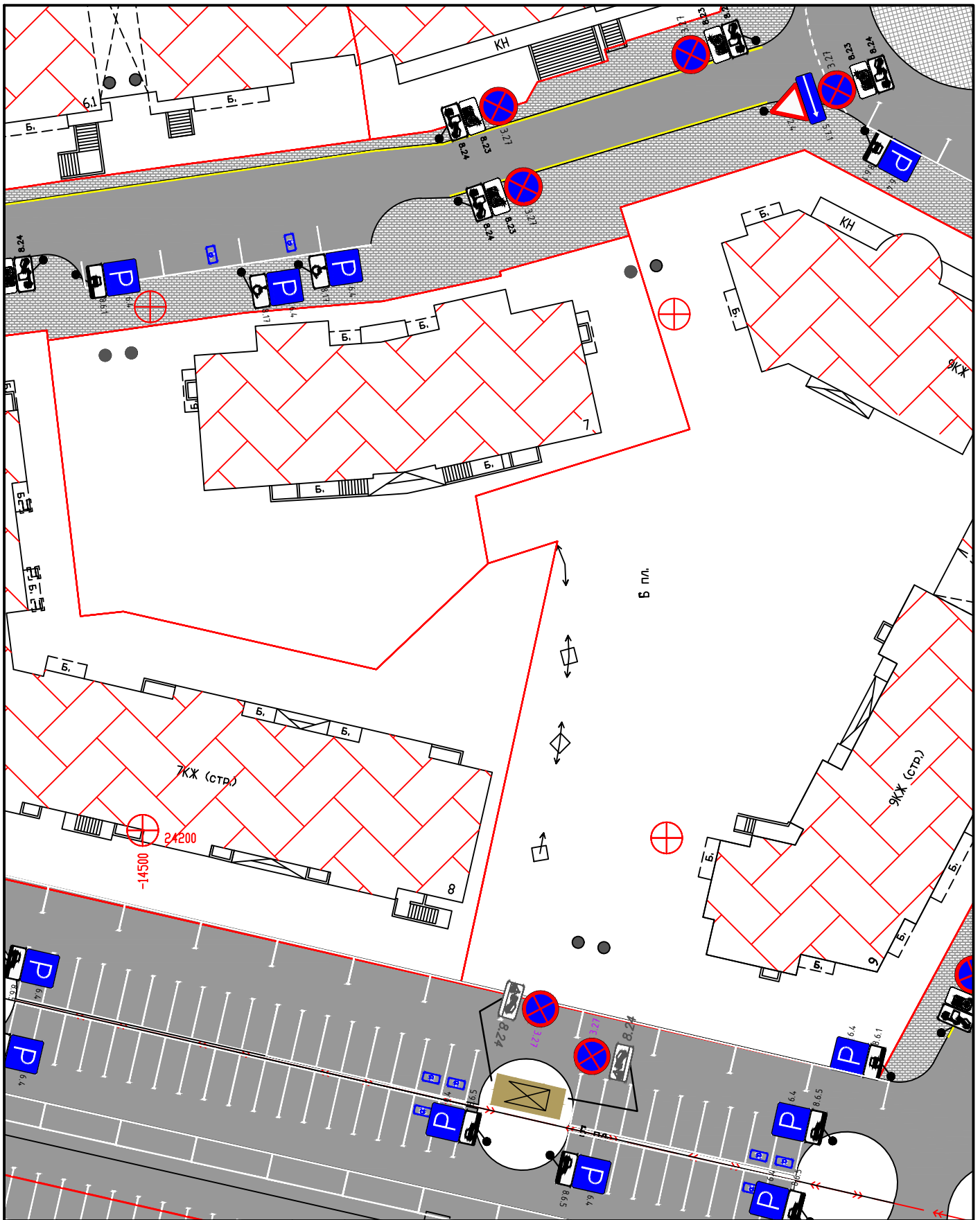
Схема организации дорожного движения вблизи д.11 по ул. Парковоя.
