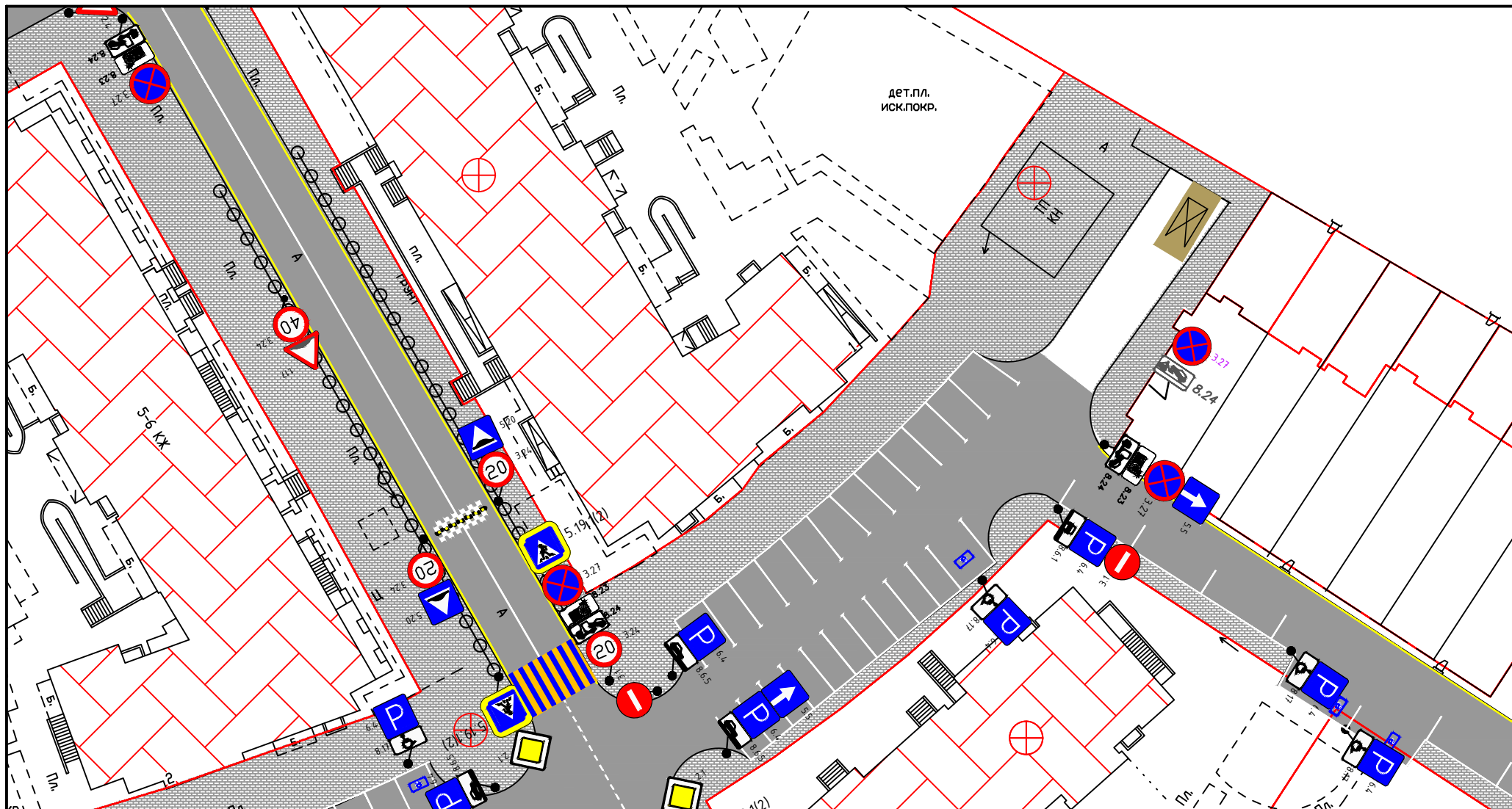
Схема организации дорожного движения вблизи д.2 по ул. Парковая.
